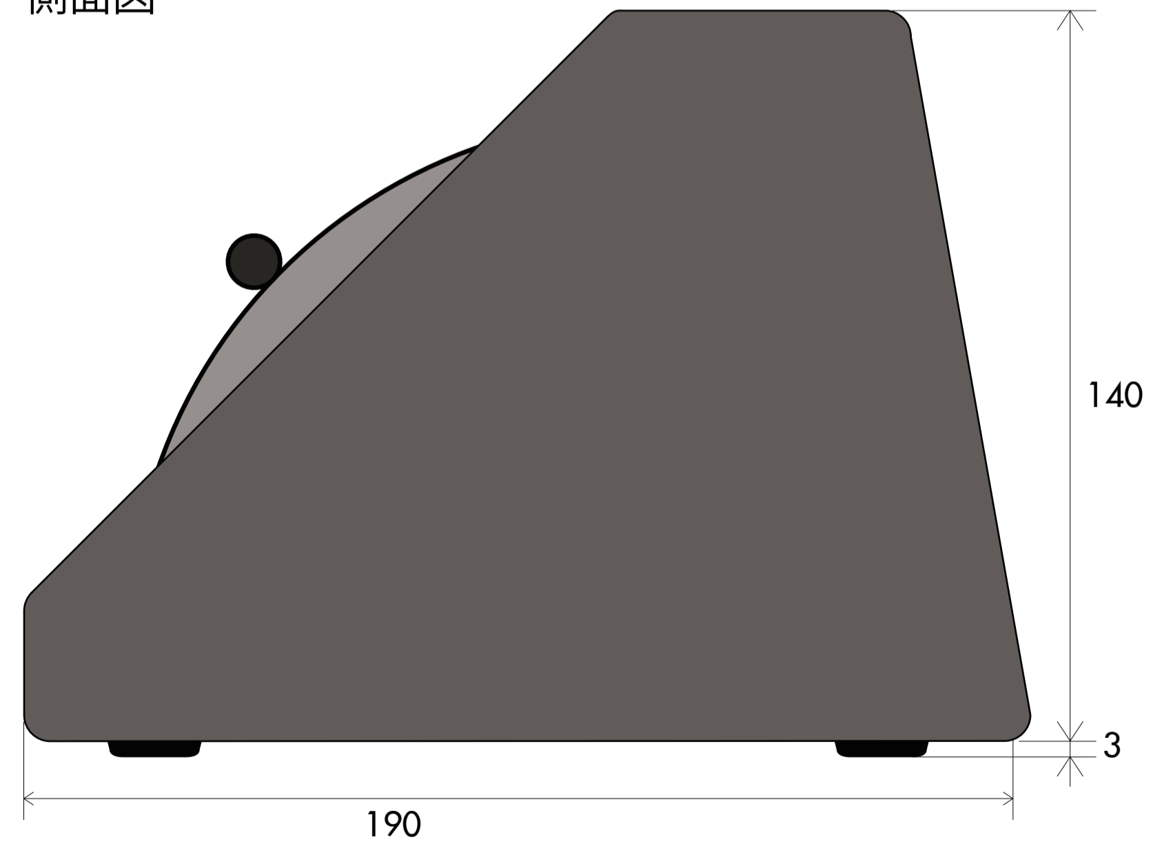
側面図
