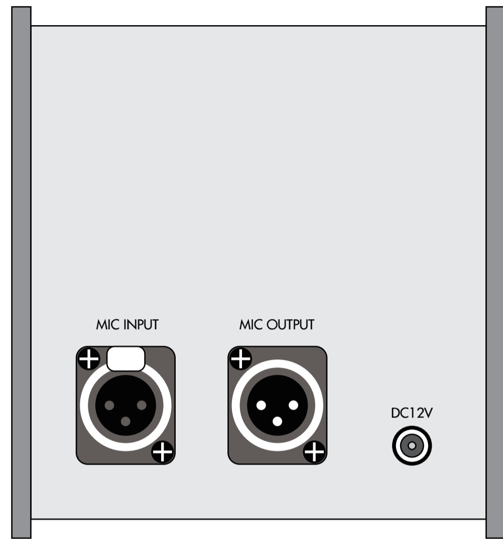
背面図
