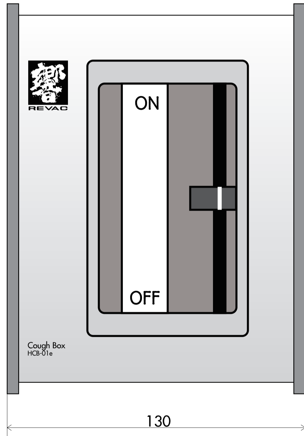
操作面図
